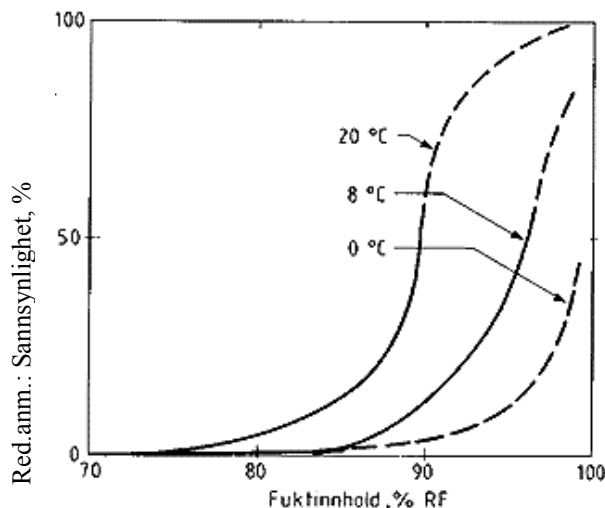
Figur 3.6—1 Red. anm.: Sannsynlighet for mugg på trebaserte materialer, avhengig av temperatur og fuktinnhold. (...)
