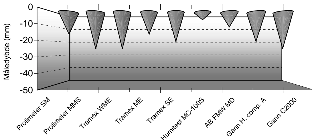
Figur 5.4—1 Vurdering av "måledybder" i trefiberplater. Utslagene avtar med dybde til fukt.
